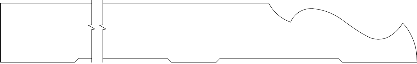
1.000" x 7.500" #1215 Base
