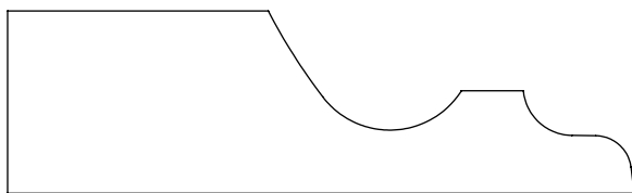
0.875" x 3.000" #1209 Base
