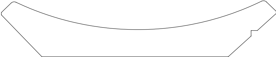
1.000" x 5.000" #4004 Crown
