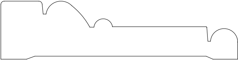
1.000" x 4.000" #2461 Casing
