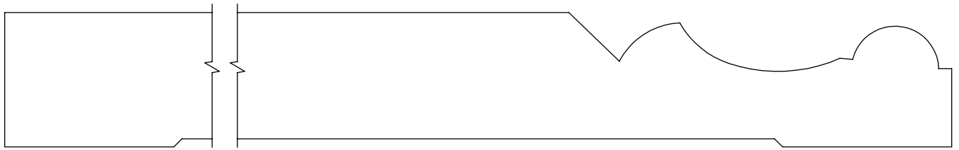
1.000" x 7.500" #1205 Base
