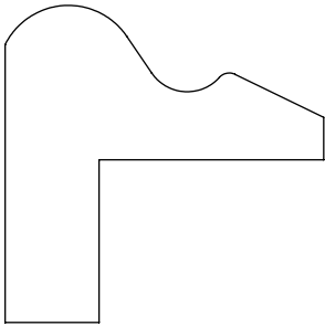
1.500" x 1.500" #3979 Backband
