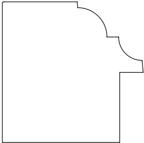
1.500" x 1.500" #3974 Backband
