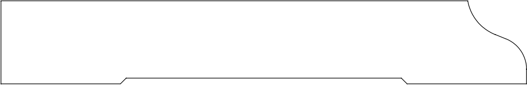
0.875" x 5.500" #1124 Base
